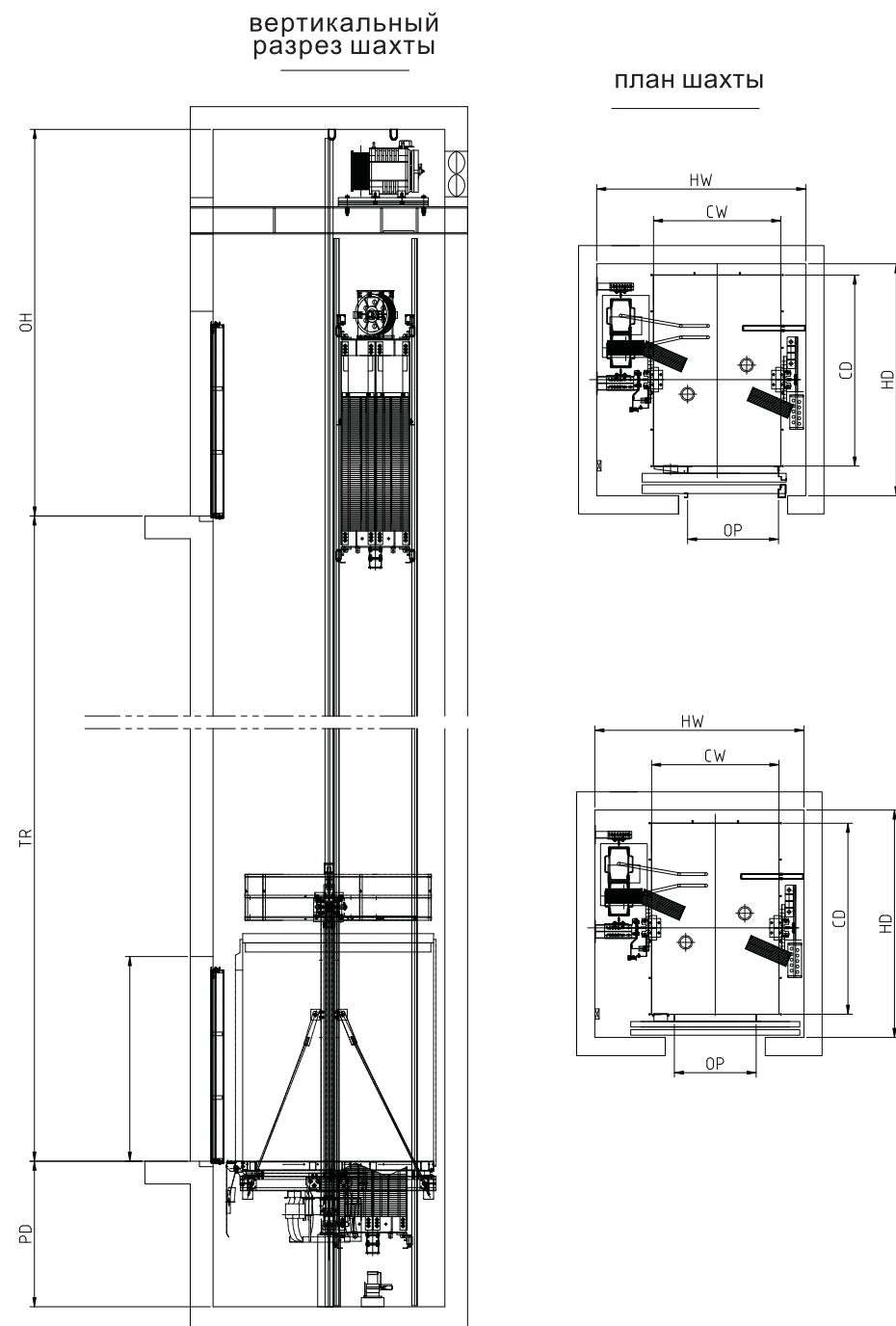
М300 (MRL) пассажирский лифт
