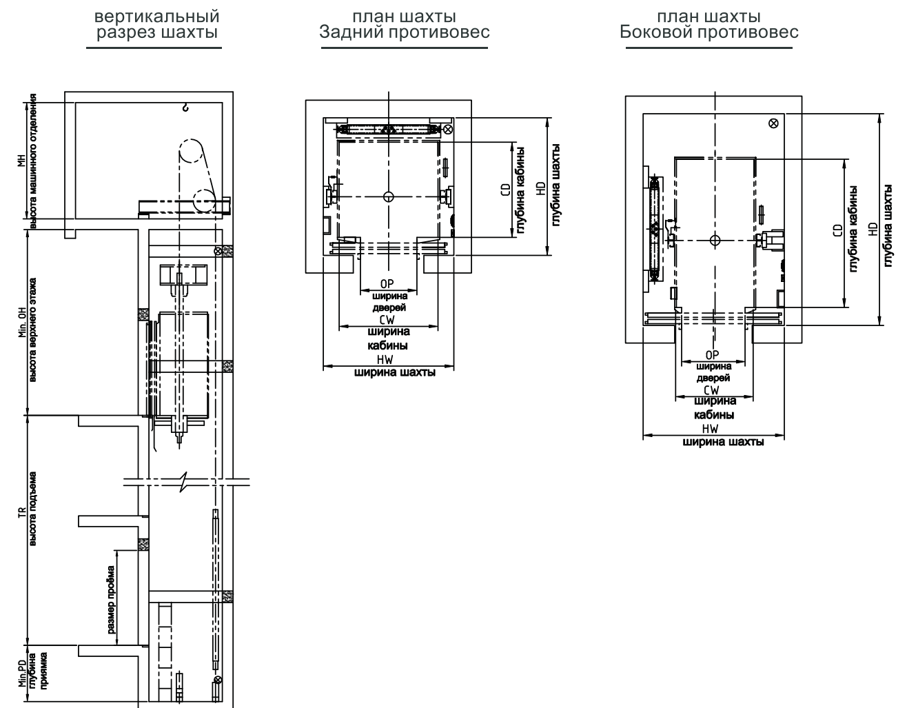
С300 (MRA) пассажирский лифт
